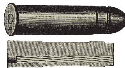
Рис. 80. Патрон для стрельбы дробинкой
