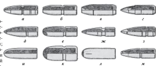
Рис. 183. Пули для нарезного охотничьего оружия: a — неэкспансивная оболочечная; б — мягкоконная с грибовидным сердечником; в — с надрезами головной части; г — с кольцевой направляющей на оболочке и отверстиями в головной части; д — с уменьшенной толщиной оболочки в головной части; е — с надрезами оболочки лепестковой формы в передней части типа «Коре—Локт»; ж — с отсутствием оболочки в задней части; з — с клином в головной части; и — с тонкостенным металлическим колпачком без пустоты в головной части; к — с надрезами и тонкой оболочкой в головной части; л — с двойной оболочкой и пустотой в головной части; м — с Н-оболочкой и пустотой в головной части, прикрытой колпачком
