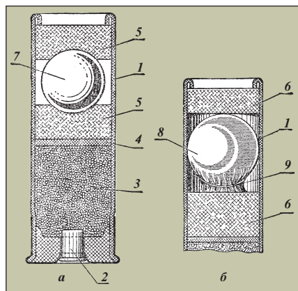
Рис. 129. Патроны, снаряженные круглыми пулями (а — центрирование пули двумя пыжами; б — центрирование пули обертыванием в замшу): 1 — гильза; 2 — капсюль «Жевело»; 3 — заряд дымного пороха; 4 — картонная прокладка; 5 — войлочные пыжи с углублениями; 6 — войлочные пыжи; 7 — круглая пуля уменьшенного калибра; 8 — пуля, обернутая в замшу; 9 — нитка
