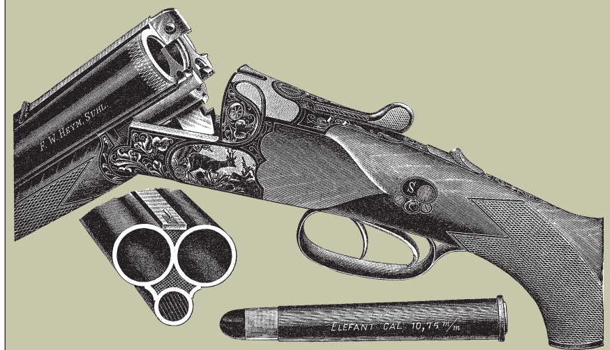
Рис. 75. Тройник с внутренними курками немецкого мастера Хэйма в Зуле. Верхние стволы дробовые, калибр 12 и 16, сверловка чок; нижний нарезной 10,75-мм
