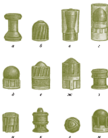
Рис. 128. Пули для гладкоствольного оружия: а — Блондо; б — Фостера; в — «Кировчанка»; г — Полева; д — шаровая; е — Бреннекс; жс — ВВОО-Ильина; з — «Идеал»; и — дважды турбинка «Майера»; к — братьев Соколовых (БС); л — «Спутник»; м — «Вятка»
