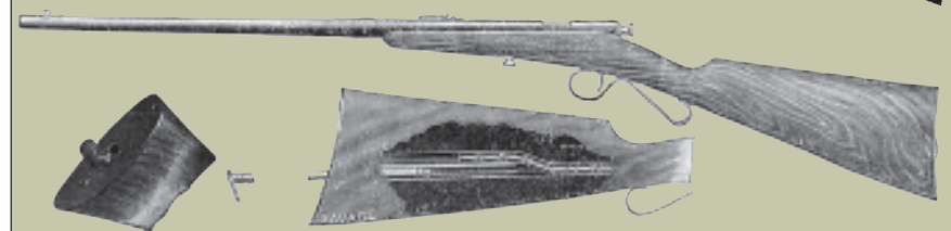
Рис. 60. Малокалиберная винтовка Сэвэдж образца 1911 г.
