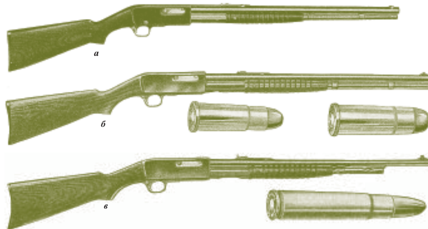
Рис. 28. Винтовки системы Ремингтон: а — образец 14 1 / 2 ; б — образец 14 1 / 2 А; в — карабин образца 14 А
