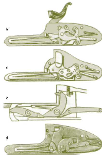
Рис. 119. Ударные механизмы: а — типа «Блиц» в ружье фирмы «Братья Меркель» в Зүле; б — замок типа Голланд—Голланд; в — системы Энсона—Дилей для бескуркового охотничьего ружья; г — системы Пэрдэй для бескуркового охотничьего ружья; д — подкладной бескурковый замок
