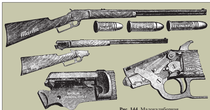
Рис. 144. Малокалиберная винтовка Марлин образца 1897 г.
