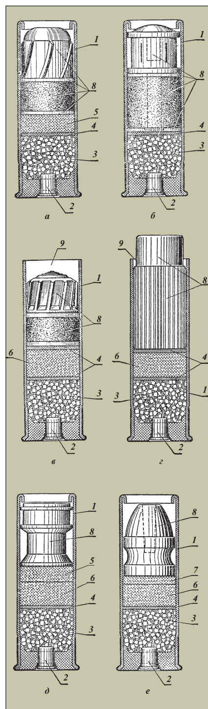
Рис. 130. Патроны, снаряженные пулями Якана (а), Ширинского-Шахматова (б), Бренке модели 1935 г. (в); Вицлебена старого образца (г), Штеденбаха модели «Идеал» (д), цилиндрической для стрельбы из ружья парадокс (е): 1 — гильза; 2 — капсюль «Жевело»; 3 — заряд бездымного пороха; 4 — картонная прокладка; 5 — войлочный пыж; 6 — осаленный войлочный пыж; 7 — суконный пыж; 8 — пуля; 9 — заливка воском
