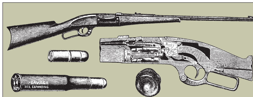
Рис. 24. Магазинная винтовка системы Сэвэдж образца 1899 г.
