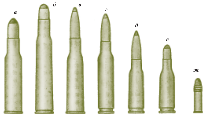
Рис. 182. Охотничьи патроны для нарезного оружия отечественного производства: a — 9×53; б — 8,2×66 М; в — 7,6×53; г — 7,62×51; д — 7,62×39; е — 5,6×39; ж — 5,5 мм кольцевого воспламенения
