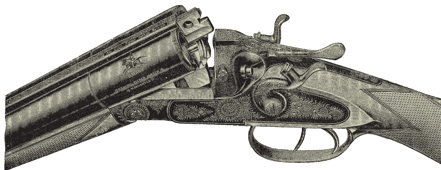
Рис. 73. Двойник «Баярд» с горизонтальным скреплением стволов
