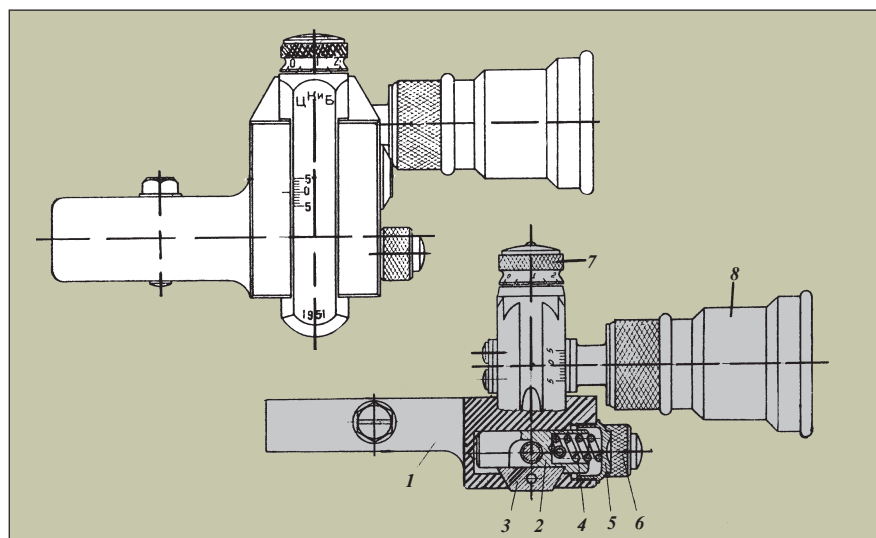
Рис. 83. Общий вид и устройство диоптрического прицела: 1 — основание прицела; 2 — корпус гайки; 3 — стойка прицела; 4 — пружина корпуса гайки; 5 — упор пружины корпуса гайки; 6 — головка тяги; 7 — головка горизонтального винта; 8 — трубка
