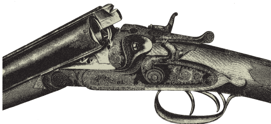
Рис. 100. Затвор системы Вестлей Ричардс
