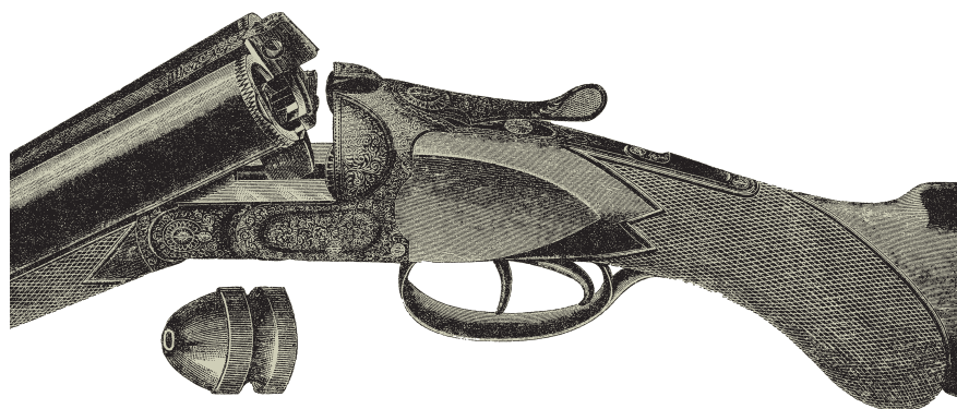
Рис. 78. Ружье-парадокс А. Франкотта 12-го калибра
