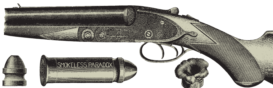
Рис. 79. Ружье «Магнум» нитропарадокс
