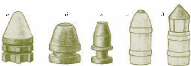
Рис. 184. Пули для оружия типа «парадокс»: a — свинцовая с медным колпачком 12-го калибра; б — свинцовая с пустотой в головной части, закрытой пластмассовой заглушкой; в — свинцовая для «парадокса» 32-го калибра «олень»; г — латунная 32-го калибра со свинцом в головной части; д — латунная 32-го калибра с алюминиевым клипом
