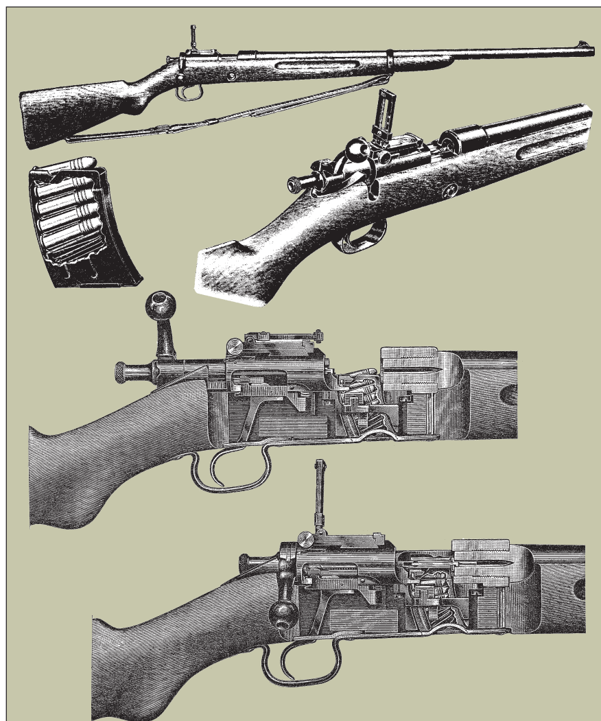
Рис. 147. Малокалиберная винтовка системы Винчестер, модель 52 и ее механизм в положении открытого и закрытого затвора
