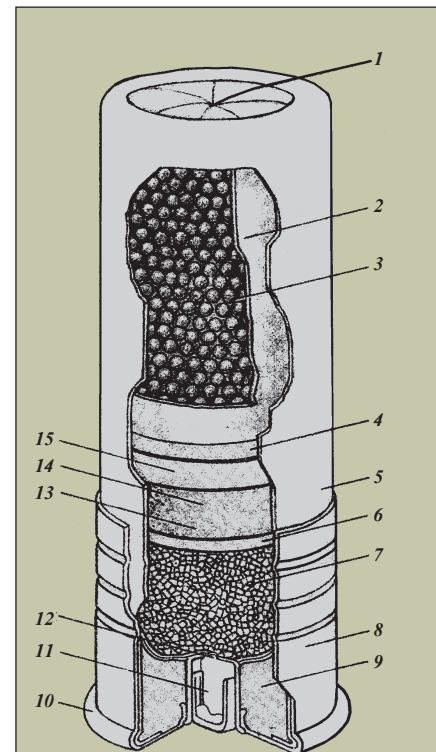
Рис. 123. Устройство дробового патрона: 1 — опрессовка «звездочкой»; 2 — контейнер (концентратор); 3 — дробь; 4, 6, 14, 15 — пыжи и прокладки; 5 — корпус гильзы; 7 — порох; 8 — основание гильзы; 9 — поддон; 10 — фланец гильзы; 11 — капсюль; 12 — запальное отверстие; 13 — осалка основного пыжа
