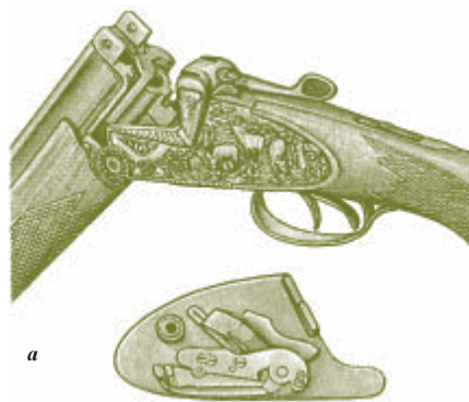
Рис. 119. Ударные механизмы: а — типа «Блиц» в ружье фирмы «Братья Меркель» в Зүле; б — замок типа Голланд—Голланд; в — системы Энсона—Дилей для бескуркового охотничьего ружья; г — системы Пэрдэй для бескуркового охотничьего ружья; д — подкладной бескурковый замок
