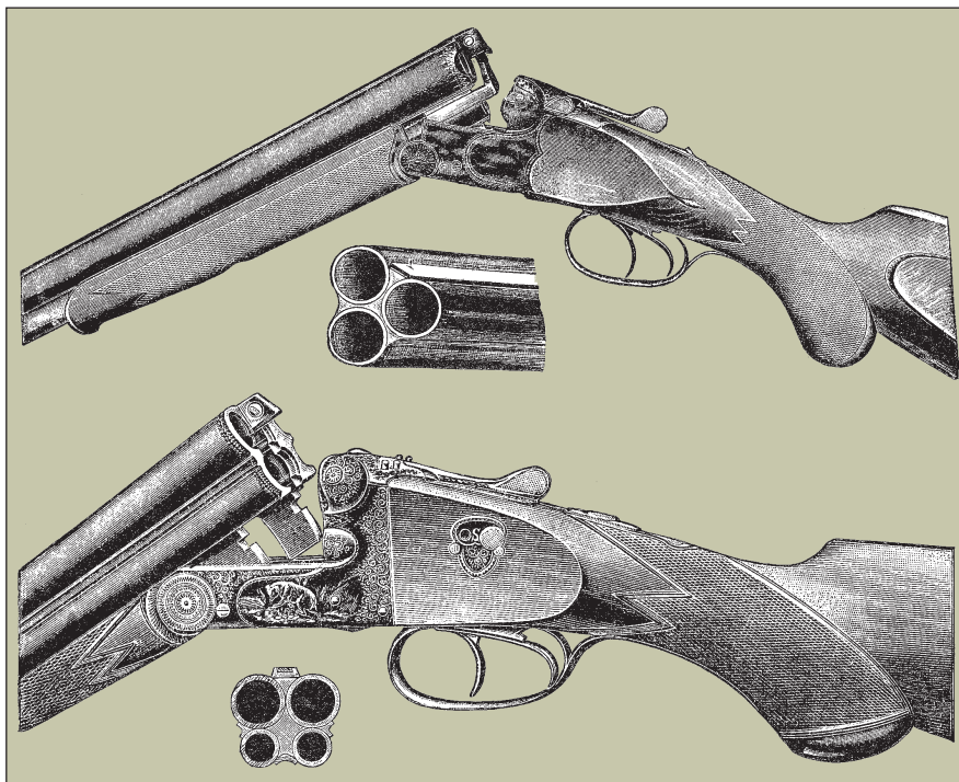
Рис. 108. Трехствольное и четырехствольное дробовые ружья германского производства
