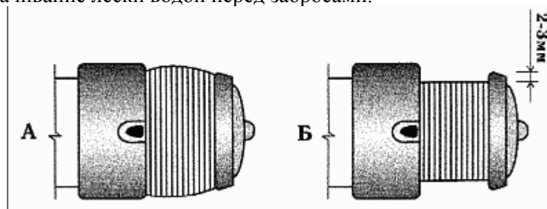
Рис. 12. «Парики» на катушках
