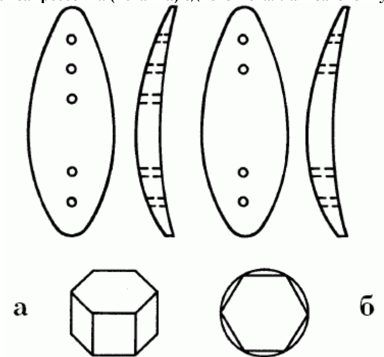
Рис. 98. Холодная запрессовка (вставка) одного металла в заготовку блесны другого
