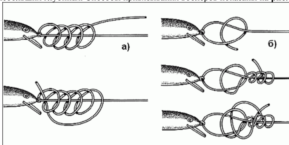
Рис. 60. Привязывание воблеров: а) с заглублением до 2 м (узел – петля); б) глубоконыряющего (жесткая фиксация на «ушке»).
