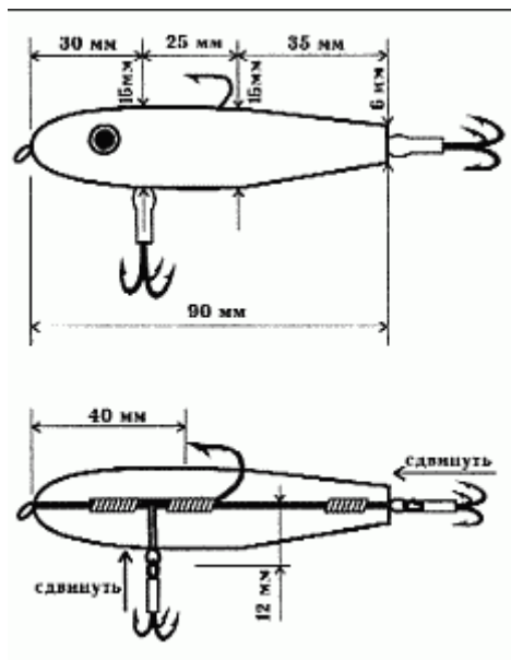
Рис. 63. Самодельные воблеры для ловли судака: а) поверхностный; б) с заглублением до 5 м
