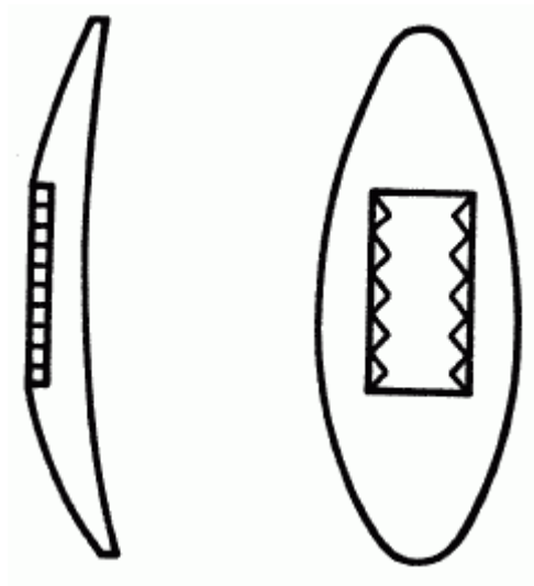
Рис. 98. Холодная запрессовка (вставка) одного металла в заготовку блесны другого
