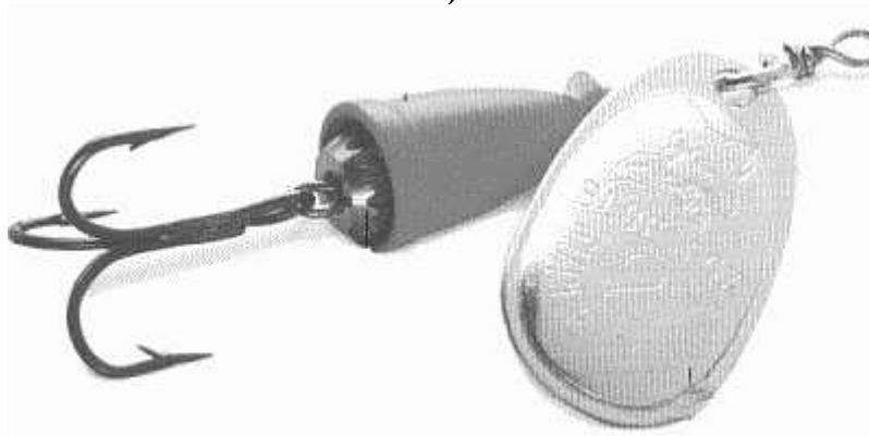
Фото 121. Акустические блесны фирмы Blue Fox: а – Vibrax Shallow для облавливания мелководных участков; б – Vibrax Original средняя глубина проводки до 1,5 метров
