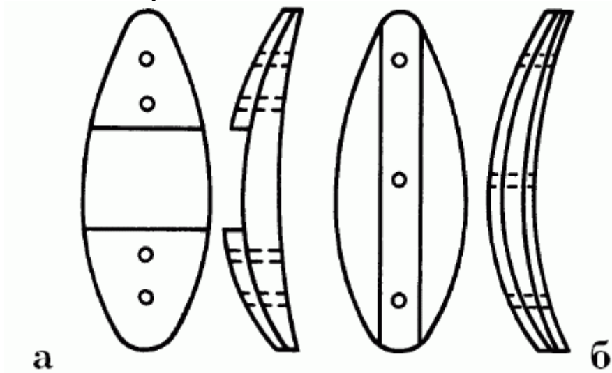
Рис. 101. Установка заклепок одного металла в заготовку блесны другого: – расположение заклепок в блесне
