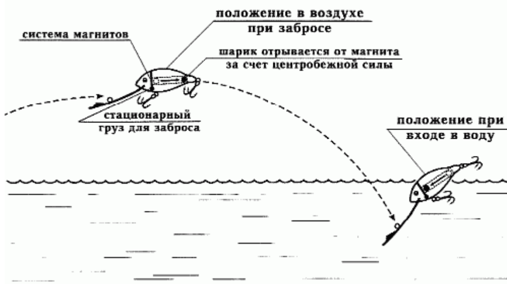
Рис. 59. Полет и «приземление» воблера с магнитной системой дальнего заброса
