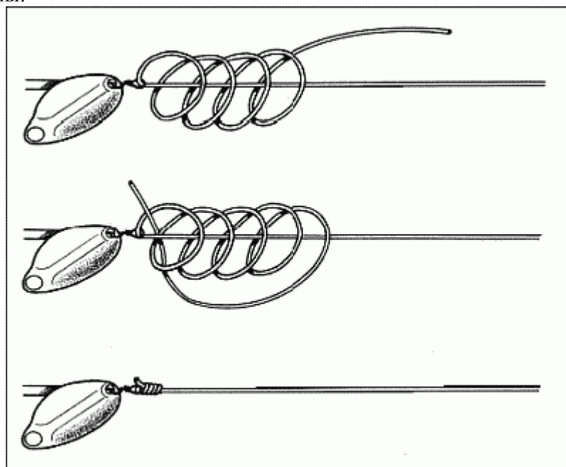
Рис. 74. Вариант привязывания вращающейся блесны Серия «Aglia»
