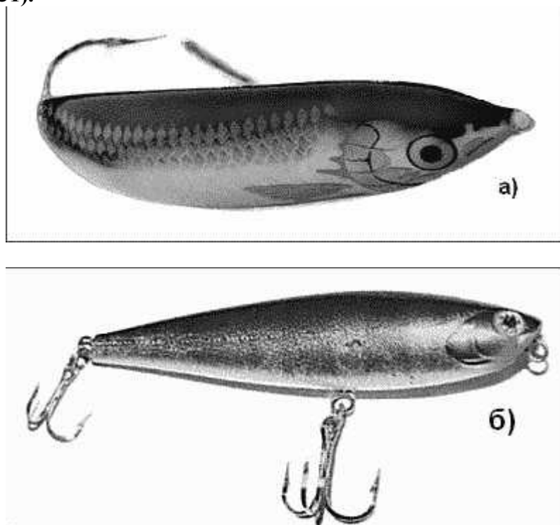
Фото 31. Безлопастные воблеры: а – Minnow Spoon с противозацепным устройством фирмы Rapala; б – Стикбейт фирмы Yo-Zori модель Arms Pensil
