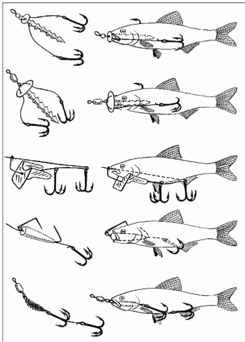
Рис. 83. Конструкции снасточек для насаживания мертвых рыбок
