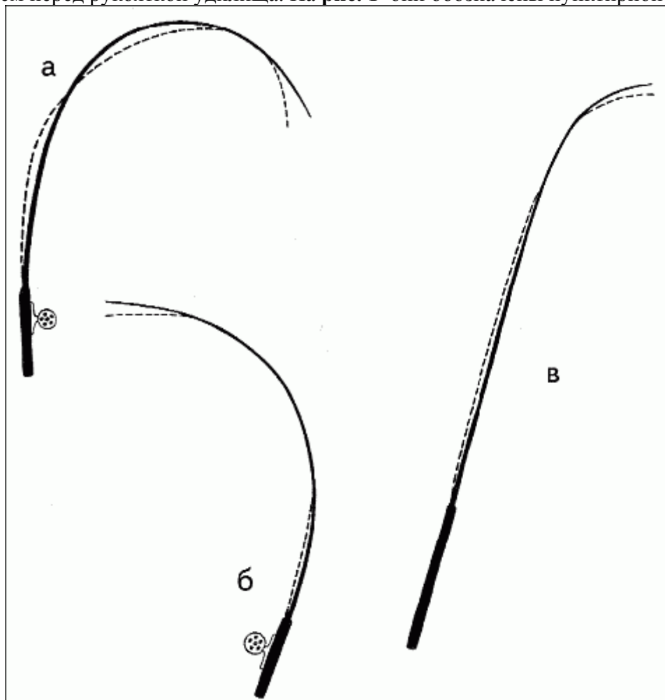
Рис. 1. Изгиб и деформации участков удилищ, обладающих сложным, комбинированным или идеальным строем: а) среднего строя при вываживании; б) среднего строя при забросе; в) сверхбыстрого строя при вываживании.
