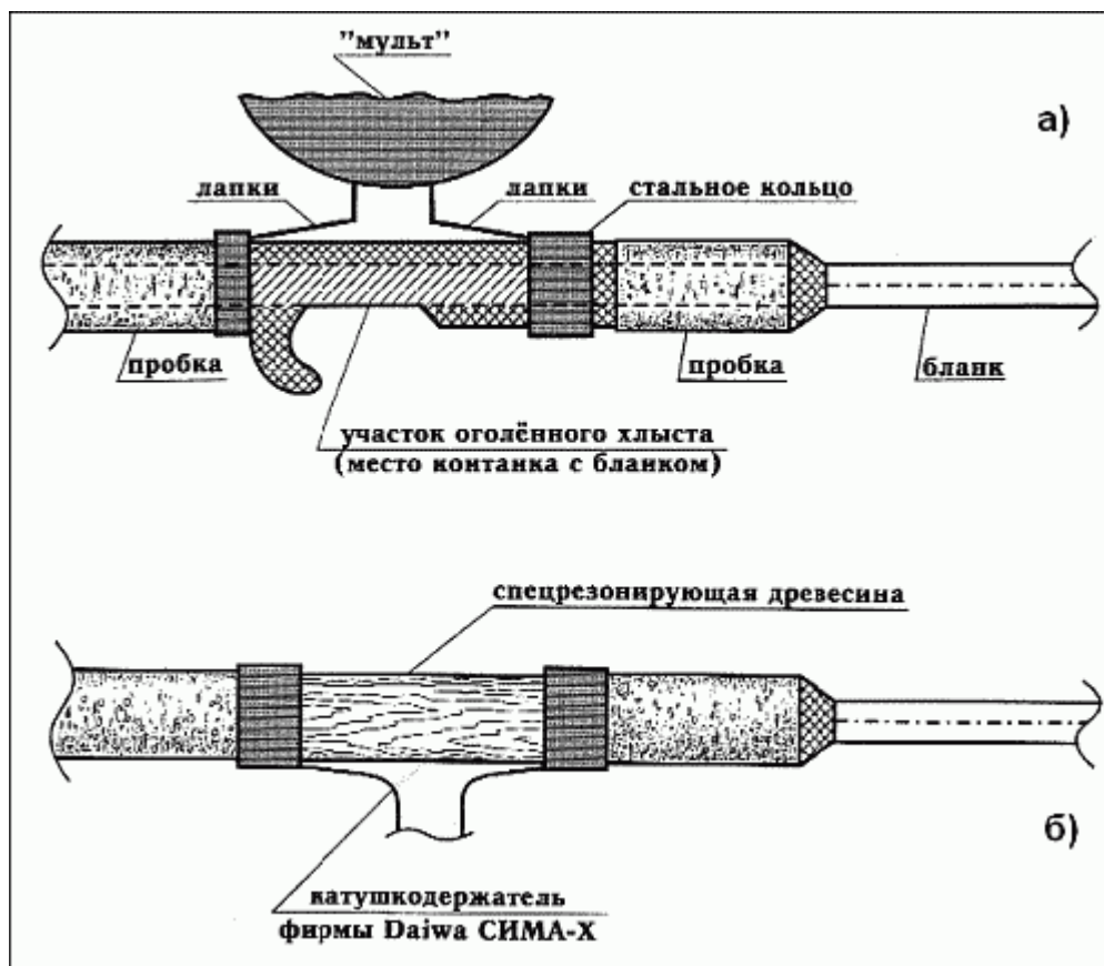
Рис. 72. Удилища с сенсорными катушкодержателями: а) под мультипликаторную катушку; б) под безынерционную.
