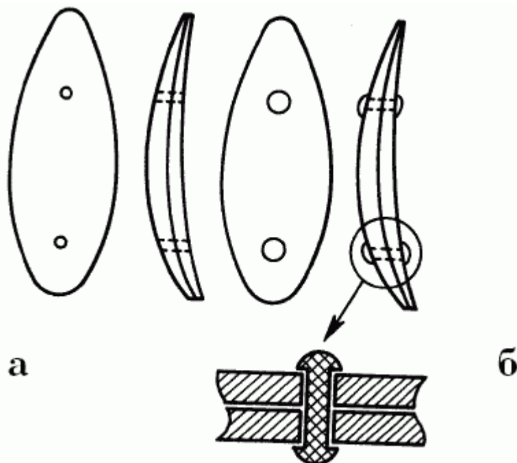
Рис. 96. Крепеж составных частей блесны на заклепках: – варианты установки заклепок
