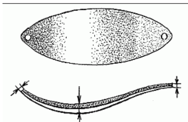
Рис. 25. Самодельная «колебалка» со смещенным центром тяжести
