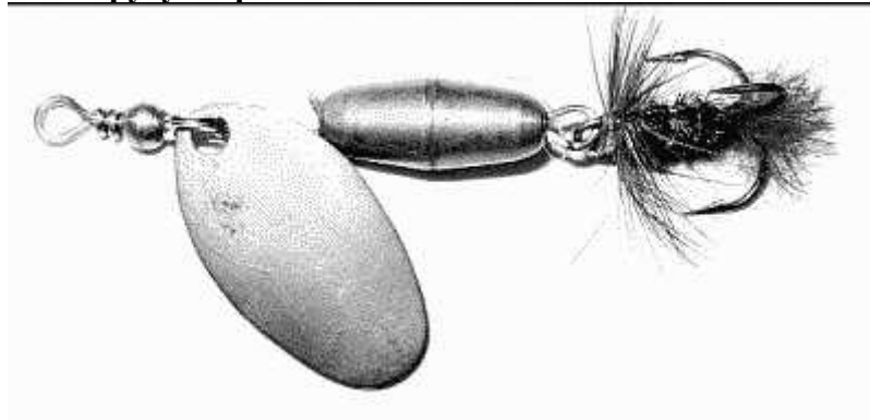
Фото 7. Микроблесны конструкции Кручинина – Моталова вес в пределах 1,2 г, угол отклонения лепестка от горизонтальной оси чуть более 30°. При всем кажущемся сходстве имеют существенные отличия в игре и прекрасно дополняют друг друга при слабом клеве. Иногда планомерная замена (через 10–15 забросов) одной блесны на другую приводит к жадной хватке хищника.
