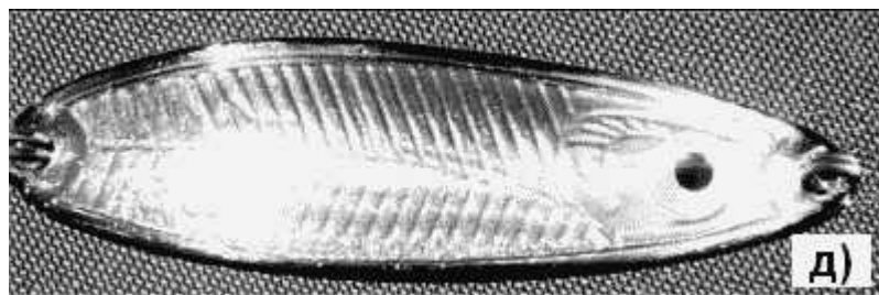
Фото 14. Колеблющиеся микроблесны: а – Palette Spoon, вес 1,5 и 2,5 г. В пластиковый корпус для баланса и веса зафиксирован металлический шарик. Изготавливается южнокорейскими фирмами по заказу фирмы TD Daiwa; б – объемная приманка Mute фирмы Jackall Bros (пластик-металл); в – блесна Mini фирмы Blue Fox. На внутренней стороне имитация икринок лосося, которые служат балансом и увеличивают дальность заброса, вес 2,5 г, длина 3 см; г – блесна Fiord Spoon (Швеция) вес 2,5 г, длина 3,2 см; д – блесна Silver Creek фирмы Daiwa, вес 3 г
