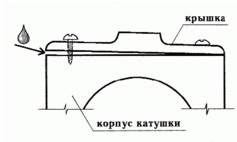
Рис. 8. Заедание катушки при вращении
