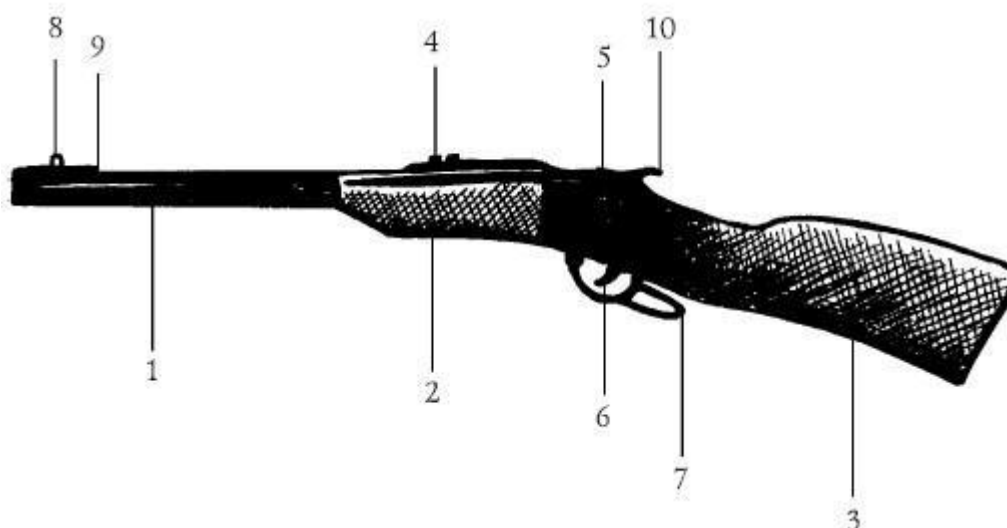
Части охотничьего ружья
